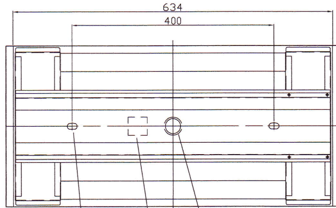
2-12X20ボルト穴 電源端子 Φ20電源穴
